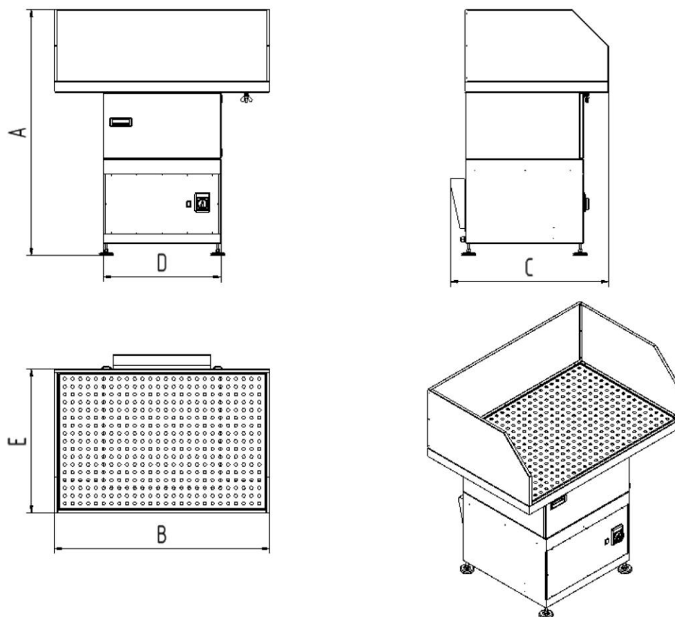
Sl. 13: List z merami
