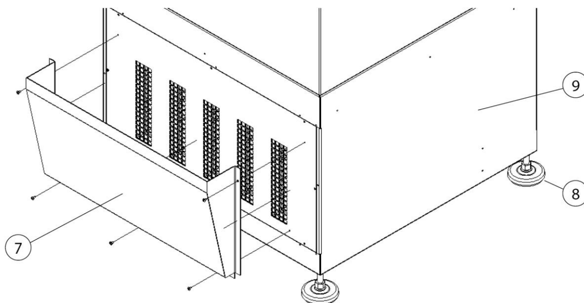
Sl. 6: Montaža izpušne lopute
